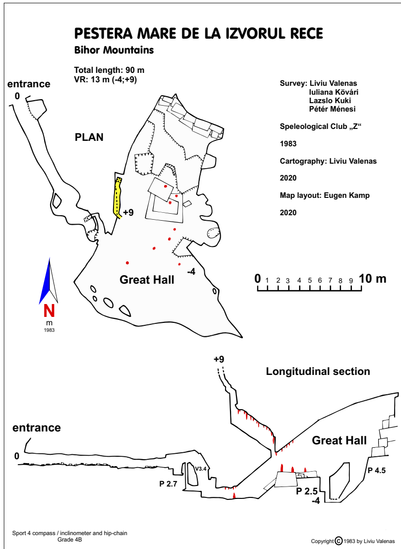
Figure 17. Peștera Mare de la Izvorul Rece, plan view by Liviu Vălenaș.
