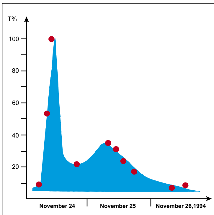
Figure 7. Graph of the tracer outpout at Izbulul Moloh (Peștera cu Apă din Cheile Someșului Cald) spring for the input in Ponorul din Cuciulata, credit by Emil Silvestru, 1995
